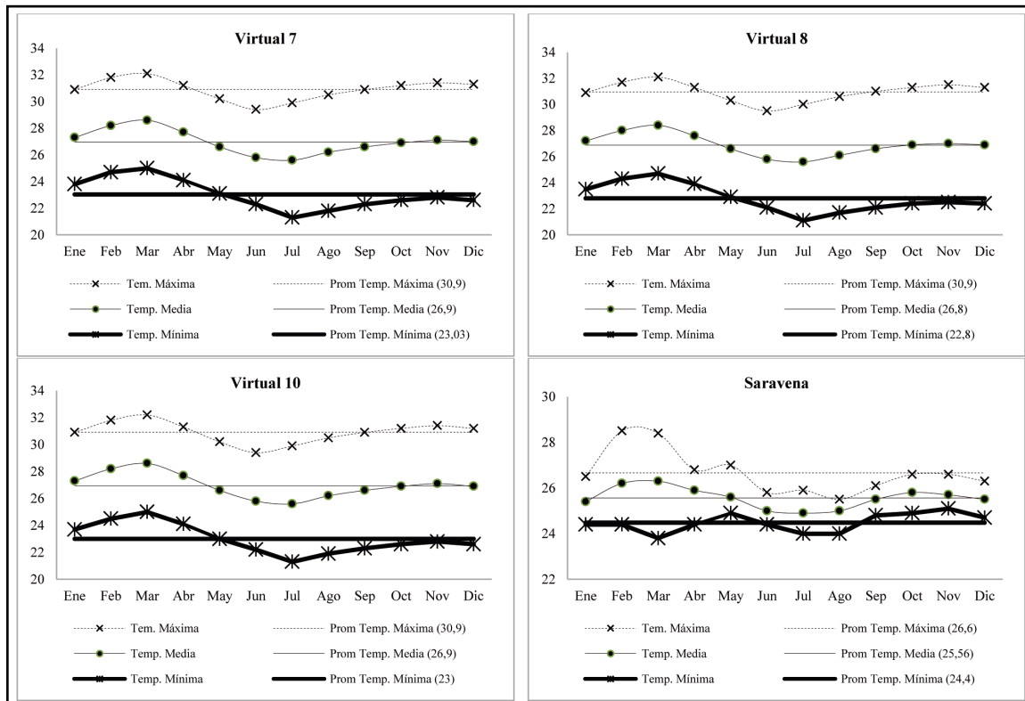
Figura 14. Variación de la temperatura máxima, media y mínima en las estaciones de la zona de estudio.
