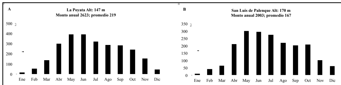
Figura 4. Balance hídrico en las estaciones de la zona de estudio.
