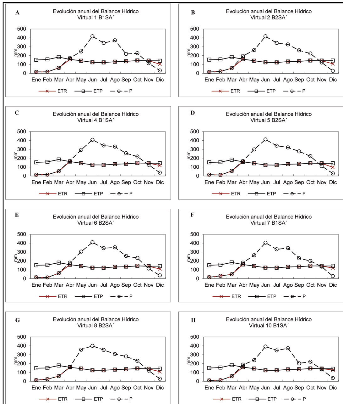
Figura 12. Balance hídrico en las estaciones de la zona de estudio.
