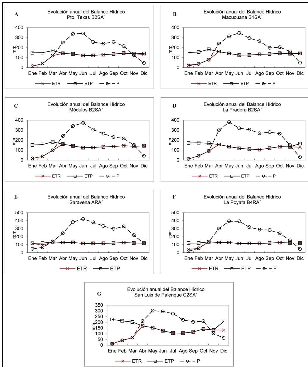
Figura 13. Balance hídrico en las estaciones de la zona de estudio.
